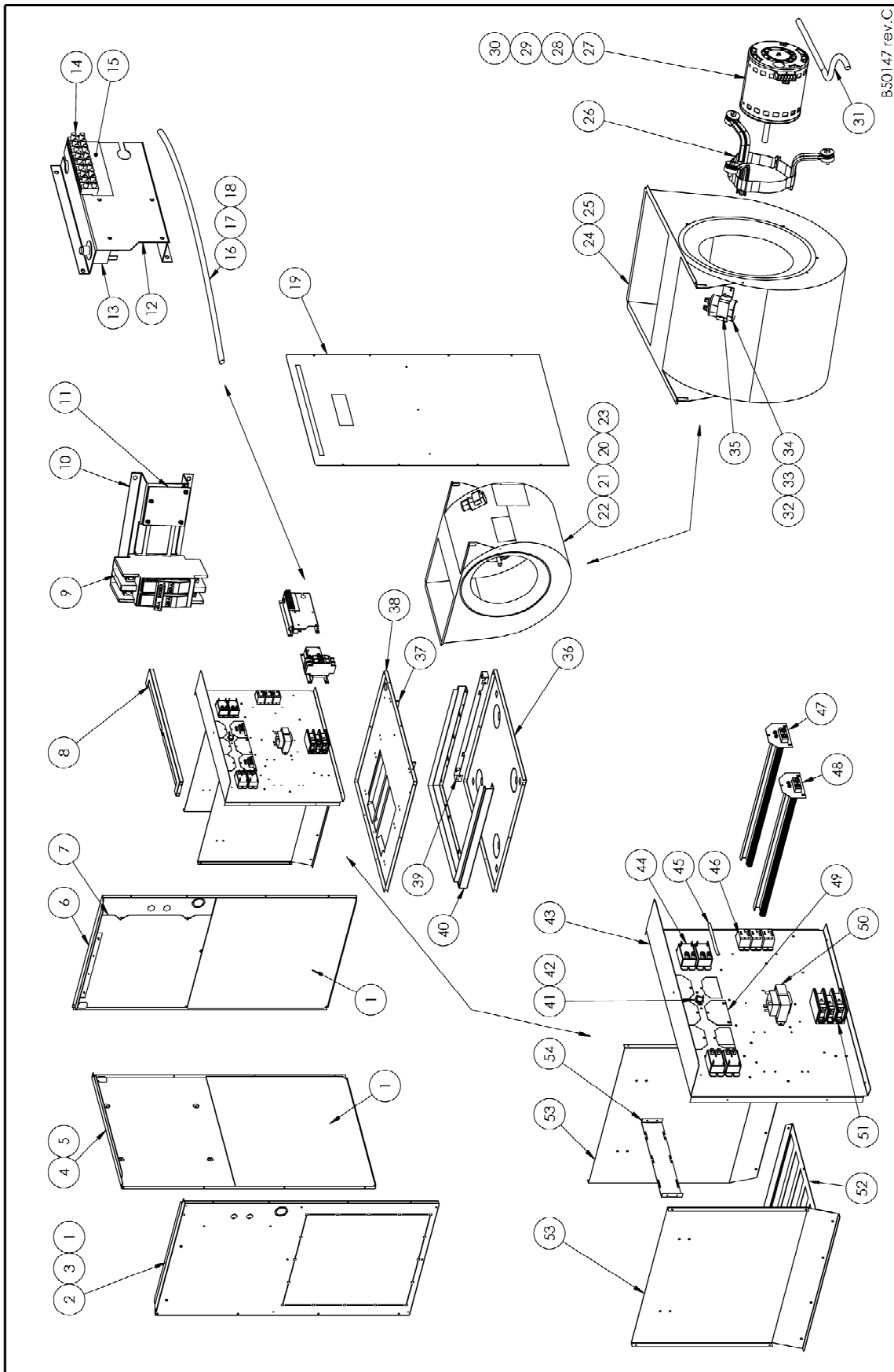
Figure 14 : Liste de pièces, SUPRÊME Confort PSC
