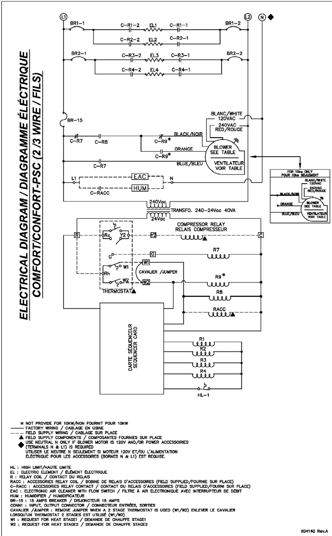
Figure 12 : Diagramme électrique, SUPRÊME Confort PSC
