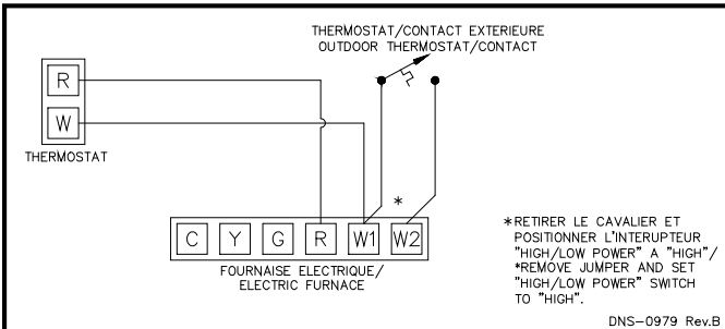
Figure 7 : Thermostat 1-stage avec contrôle extérieur pour fonctionnement en mode 2-stages, chauffage électrique seulement
