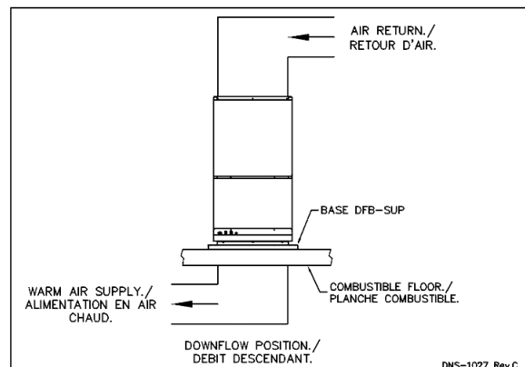
Figure 2 : Configuration, débit descendant
