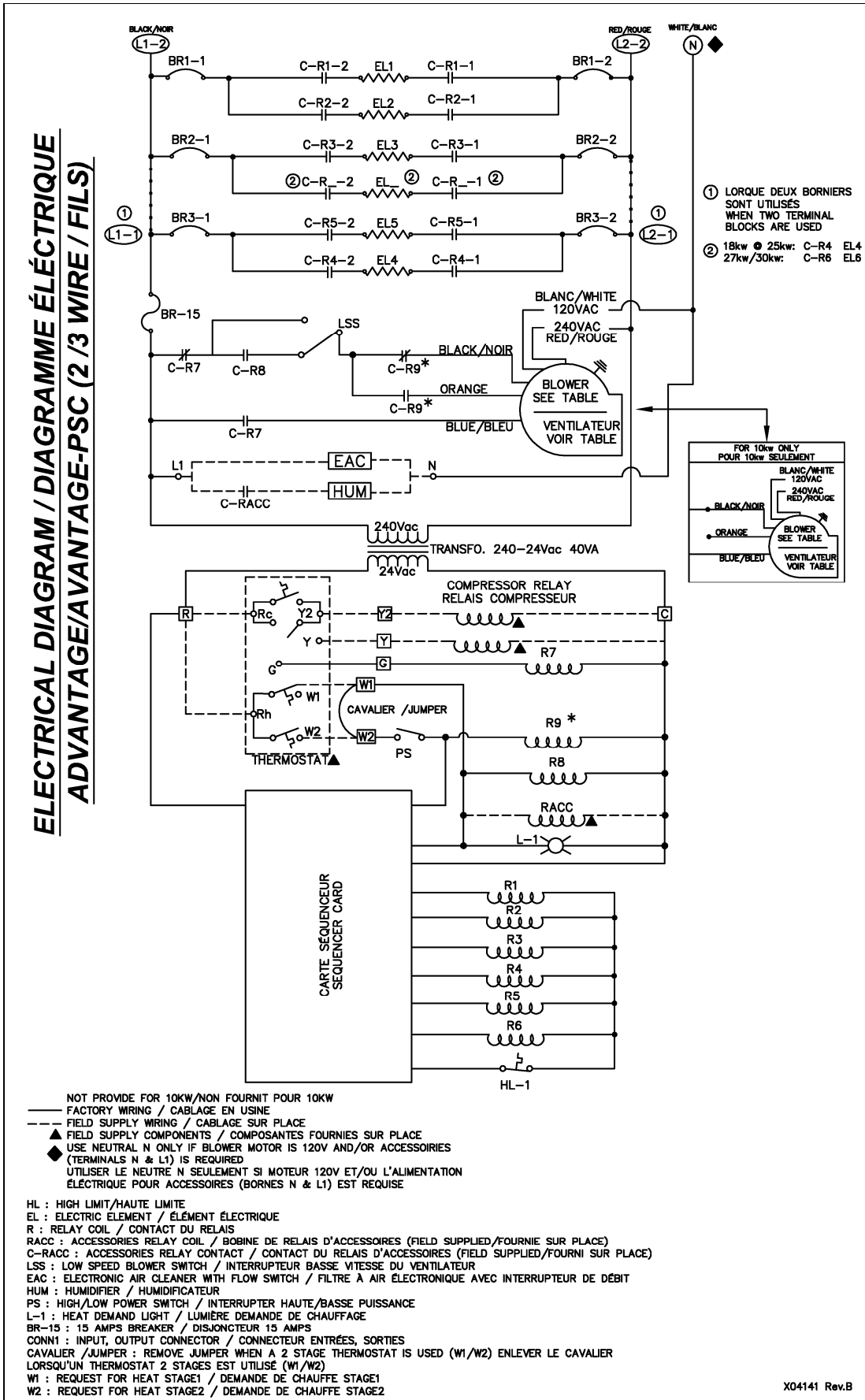
Figure 13 : Diagramme électrique, SUPRÊME Avantage PSC
