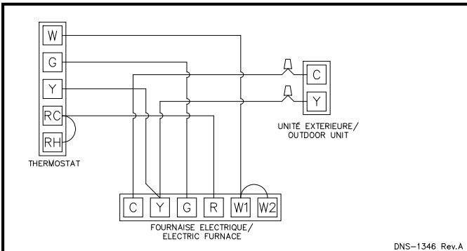
Figure 8 : Thermostat 1-stage, chauffage électrique et climatisation
