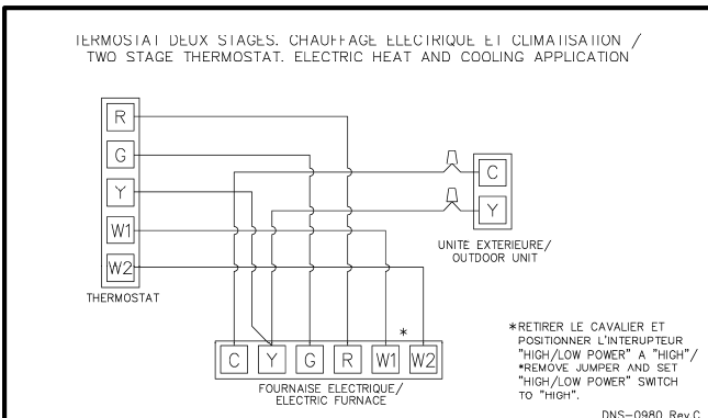
Figure 9 : Thermostat 2-stage, chauffage électrique et climatisation
