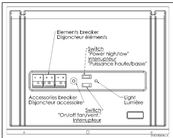
Figure 10 : Commandes sur la fournaise Advantage
