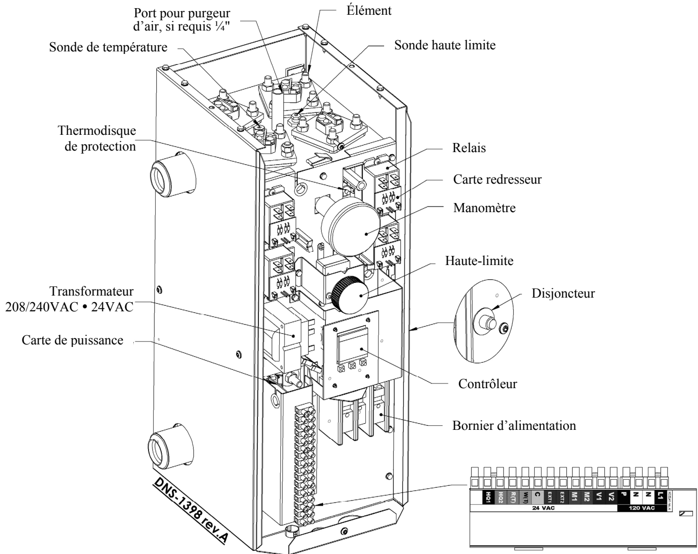
Figure 2: Composantes de la chaudière
