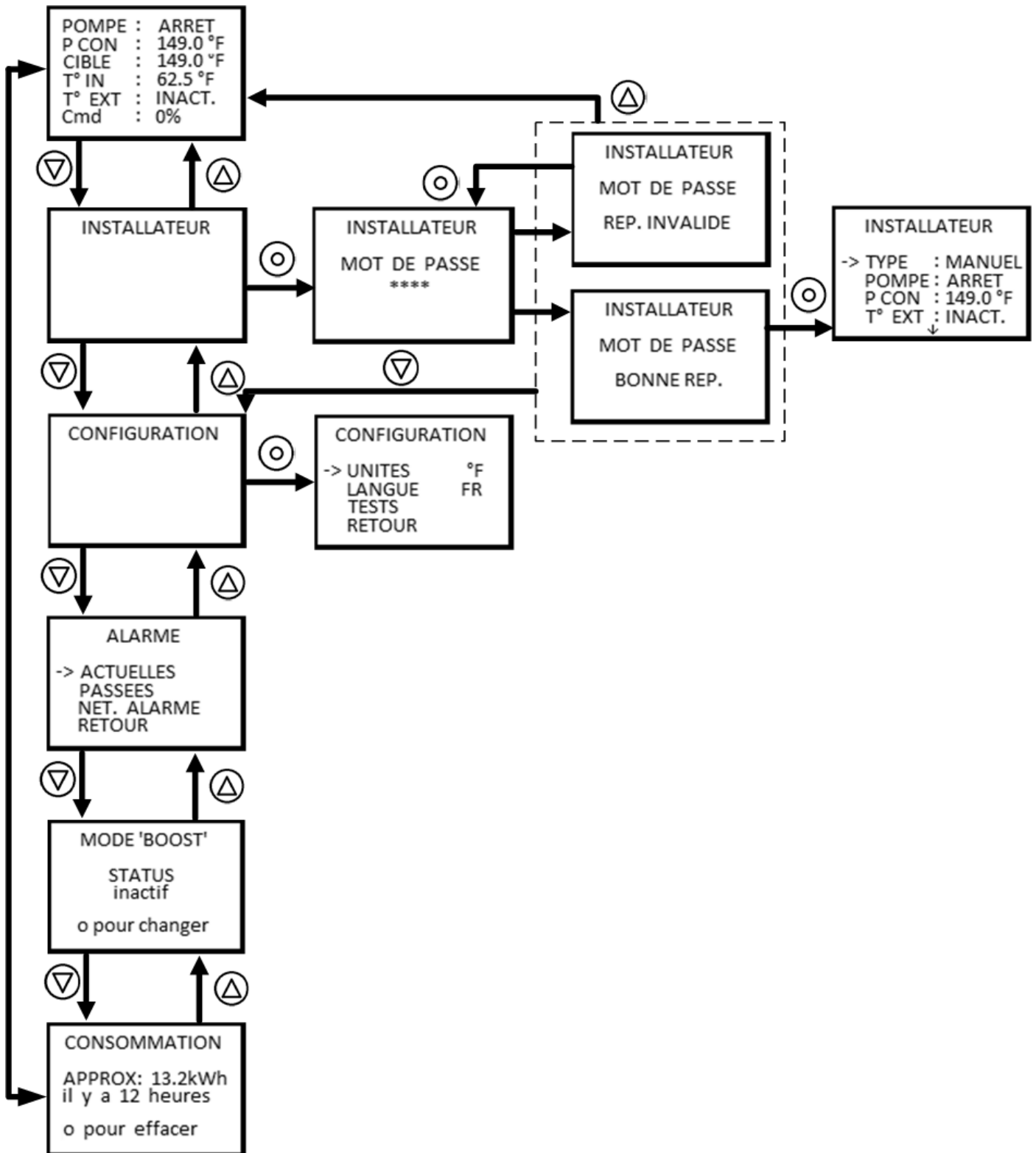
Figure 4: DÉPLACEMENT DANS LES MENUS
