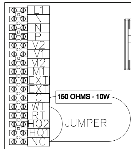
Figure 3: Résistance pour thermostat "power stealing"
