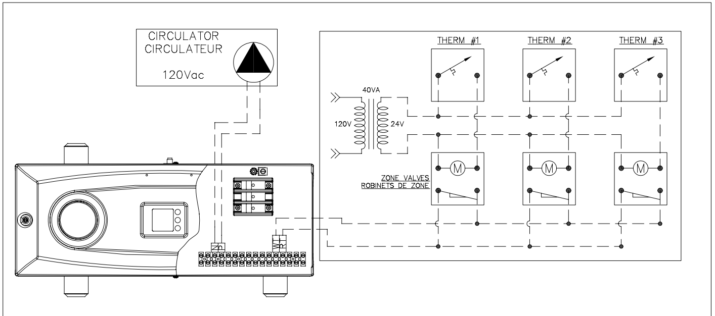
Figure 9: Diagramme multizone avec valves motorisées
