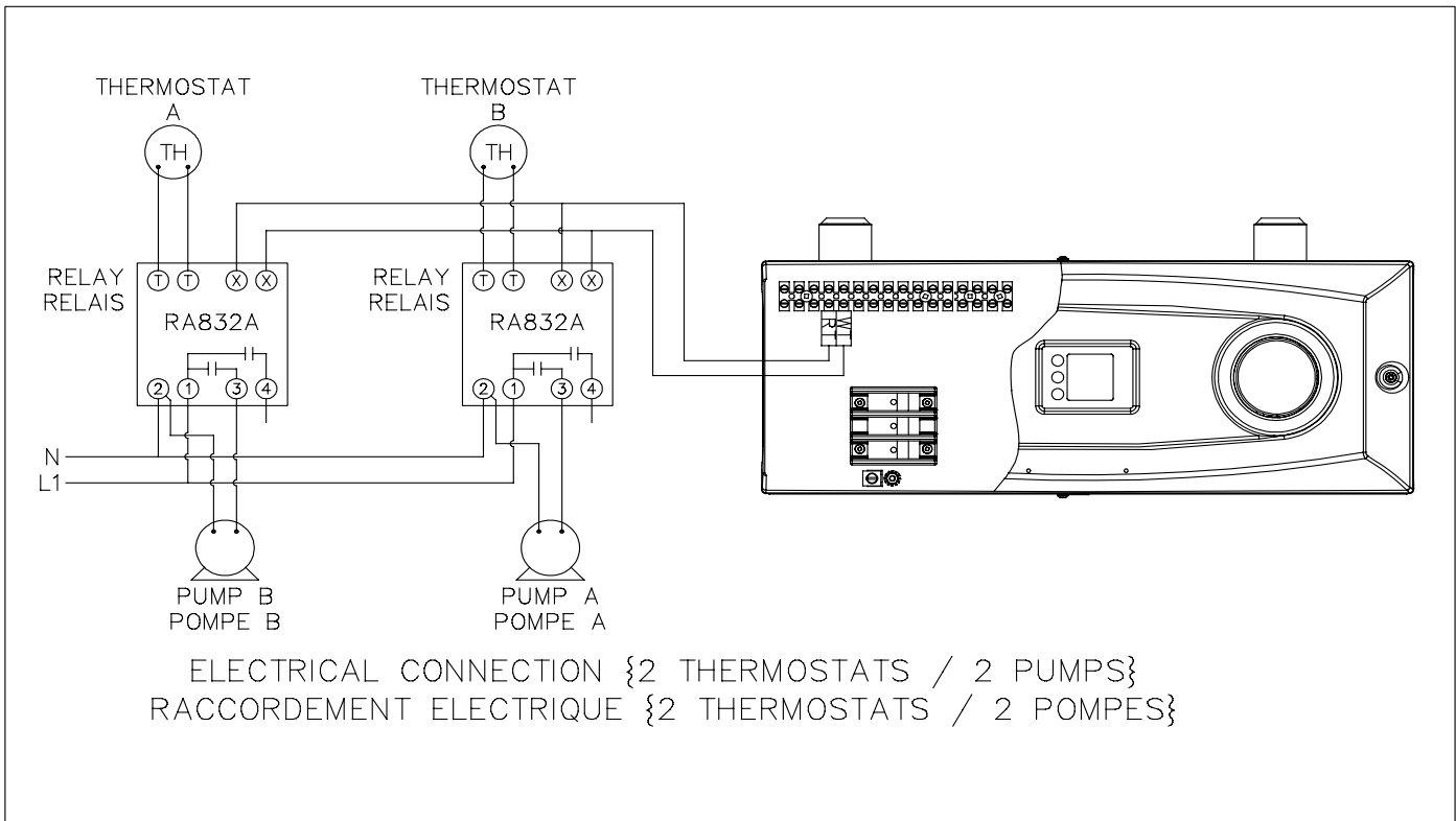
Figure 8: Diagramme multizone avec plus d'un circulateur
