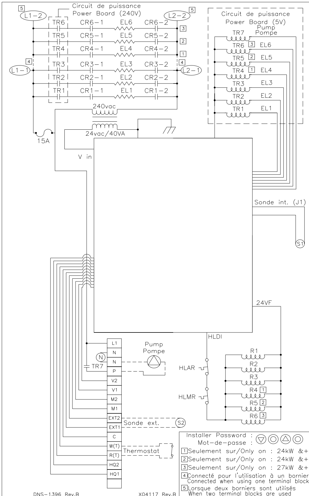
Figure 11: Diagramme électrique
